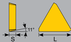
TPKN 1603
