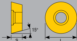
RD 12T3
