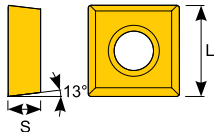
SPMG 05
