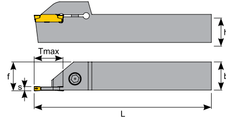
Grooving Holders
