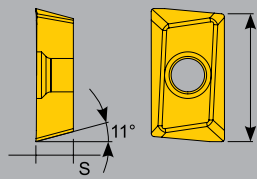
ADKT 1505
