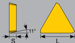
TPKN 2204
