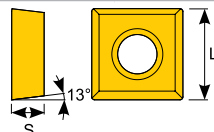
SPMG 07
