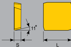
SPKN 1203
