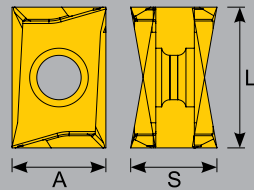
ANKX 1710
