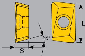
XOMX 1806
