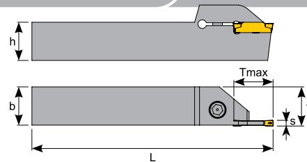
Grooving Holders
