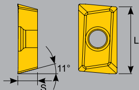
APKT 1003
